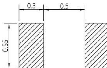
建议焊盘图
