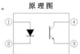
引脚配置
