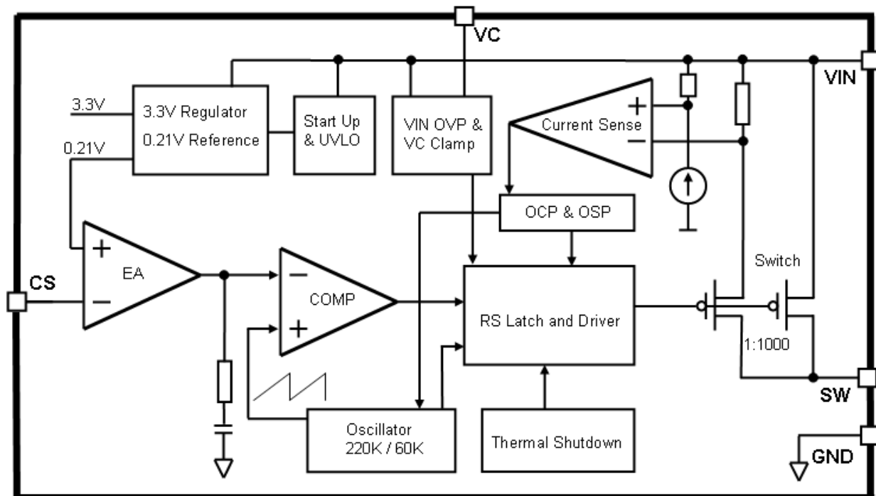
图 3. XL3005 方框图
