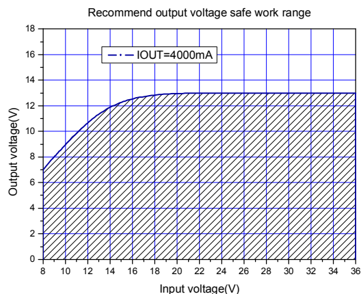
图 10.最大输出电压(IOUT=4000mA)
