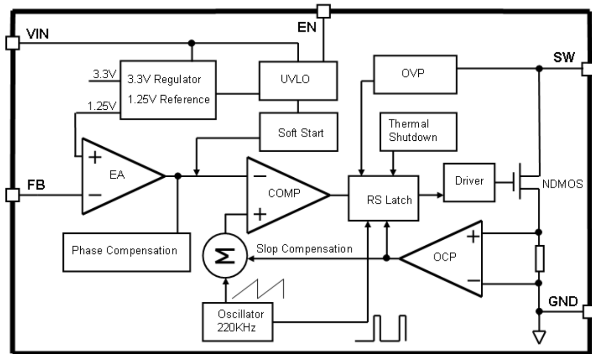
图 3. XL6019 方框图
