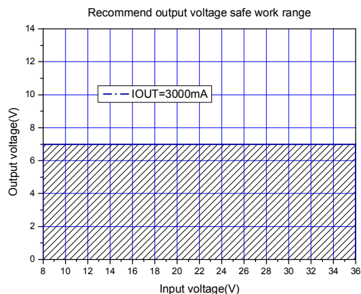
图 10.最大输出电压(IOUT=3000mA)
