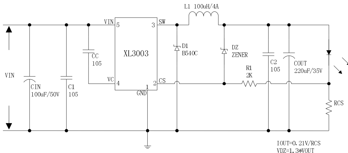
图20. XL3003系统参数测量电路（LED OVP）
