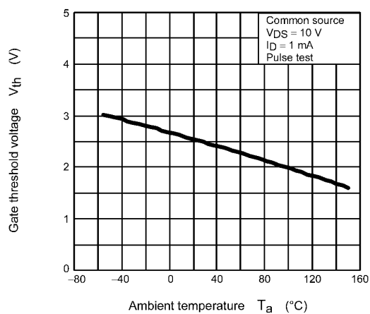
Fig. 8.10 V_{th} - T_a
