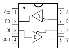
DIP/SO
