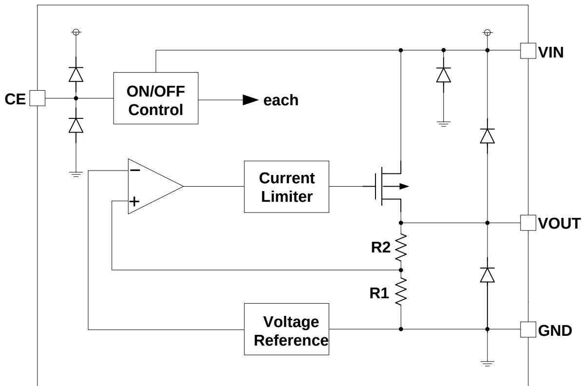
功能块框图
