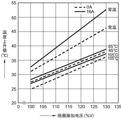
3. 线圈温度上升
