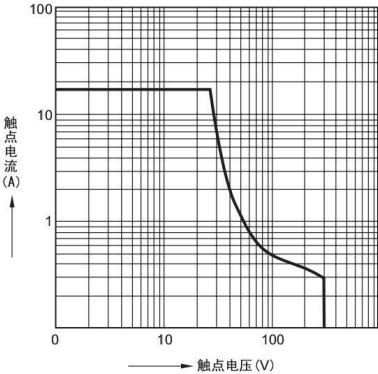
2. 通断容量的最大值 (DC电阻负载)
