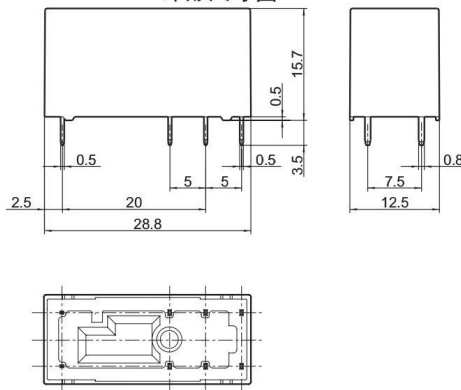
外形尺寸图
