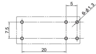
印刷电路板加工图
