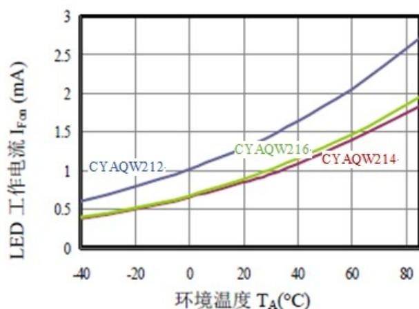
图 5: LED 工作电流-环境温度特性
