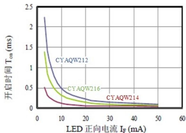
图 10: LED 开启时间-正向电流特性
