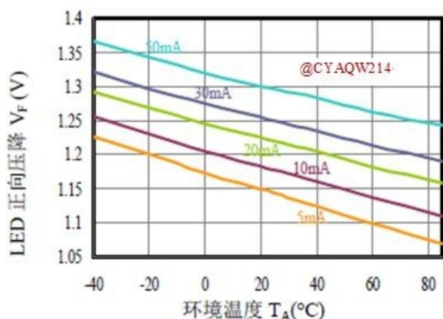
图 7: LED 正向压降-环境温度特性
