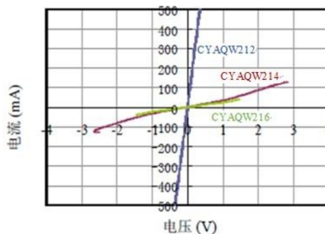
图 8: 输出端电流-电压特性
