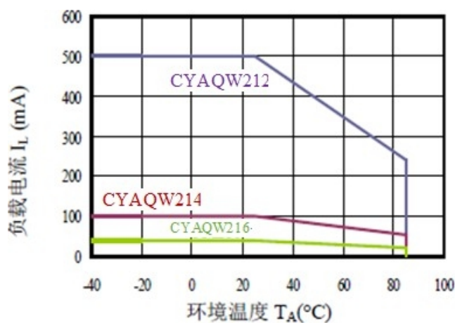
图 1: 负载电流-环境温度特性
