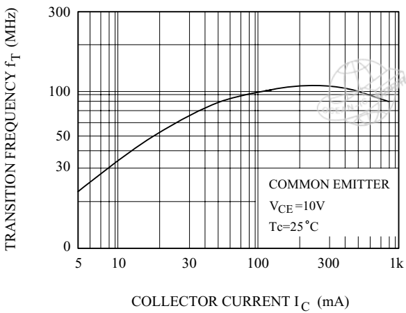
f_T - I_C
