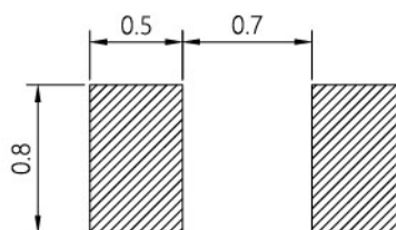
建议焊盘图
