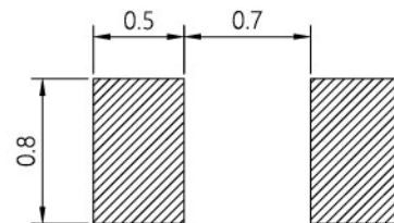
建议焊盘图
