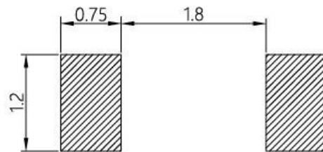
建议焊盘图
