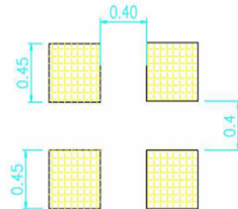
建议焊盘尺寸
