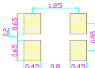
建议焊盘尺寸
