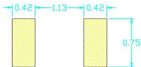
推荐焊盘尺寸
