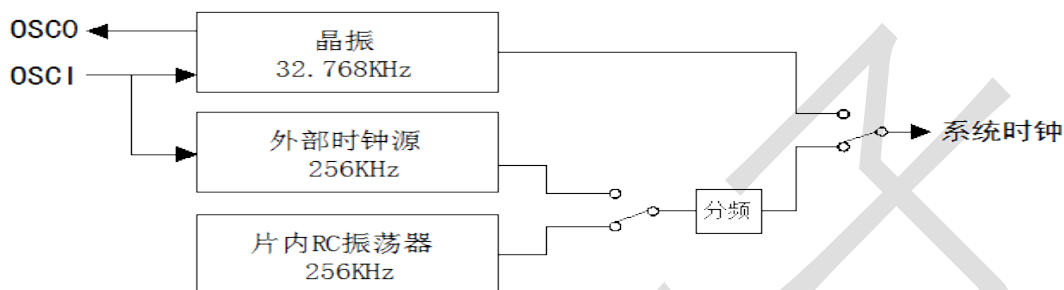
系统振荡器配置图
