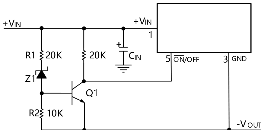
图 7. 升降压电路欠压锁定
