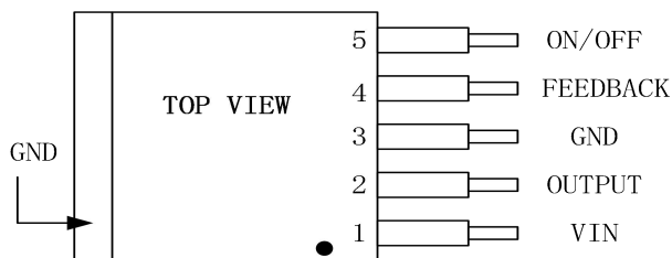
TO263-5
