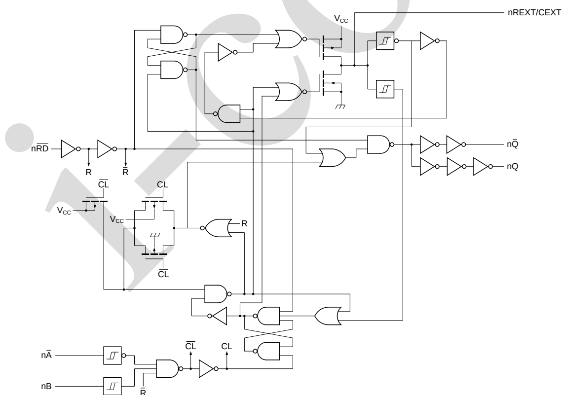
图 4 逻辑框图
