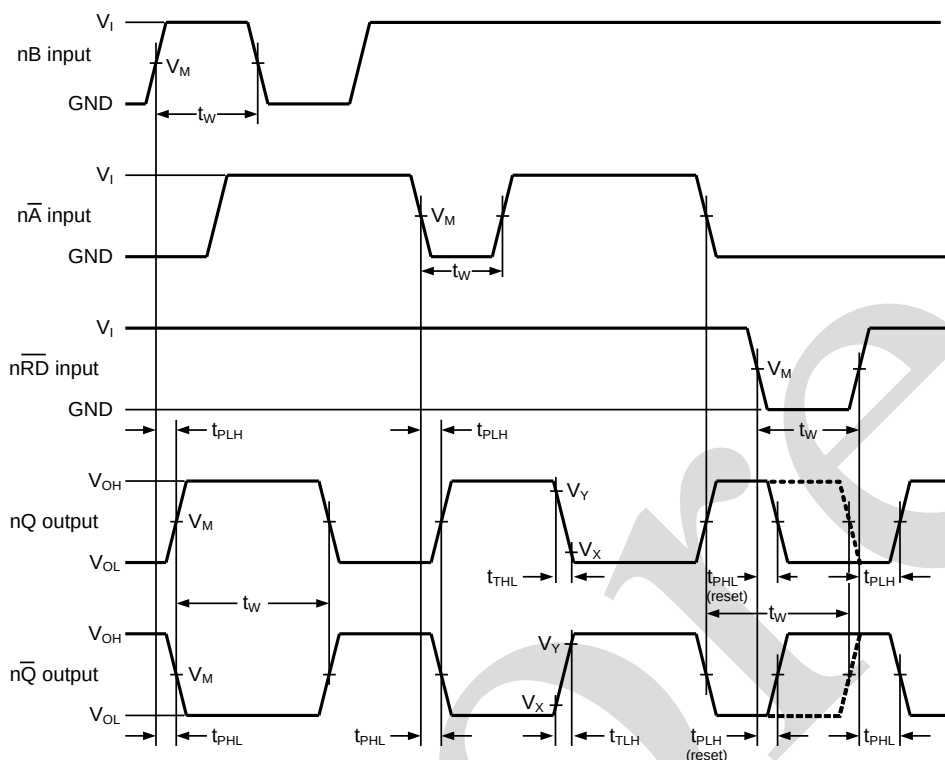
图6 输入 ( \overline{nA} , nB , \overline{nRD} ) 到输出 ( nQ , \overline{nQ} ) 的传输延时和输出转换时间
