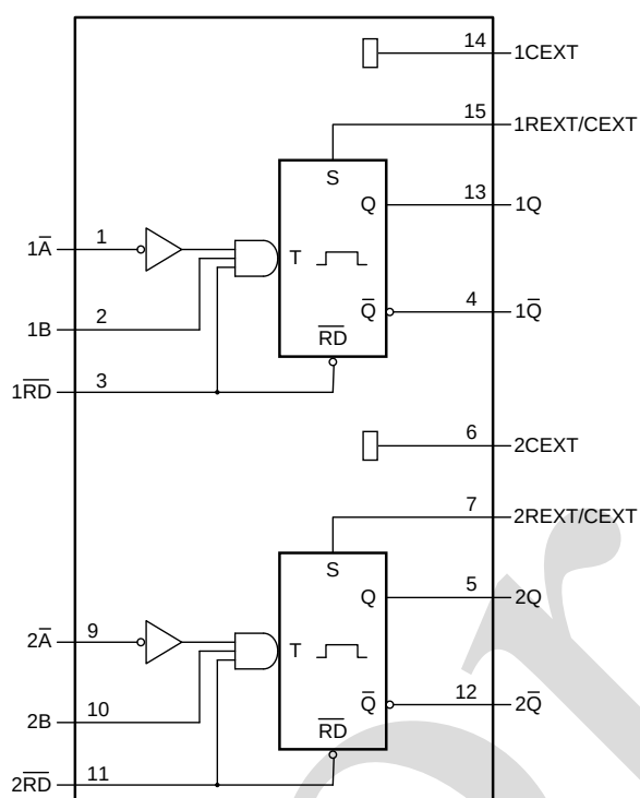
图 3 功能框图
