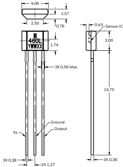
SS460-LP Sensor IC
