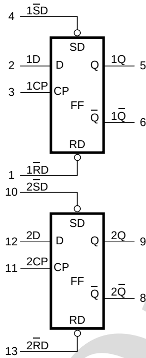
图 4 功能框图
