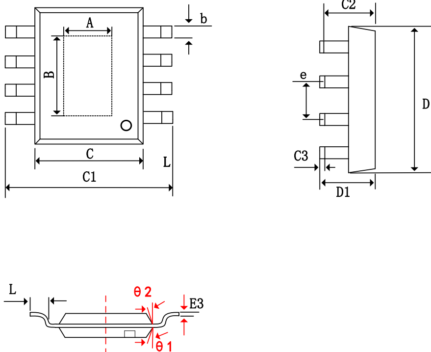
ESOP-8
