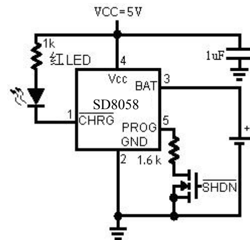
图 1：可信号控制充电电路
