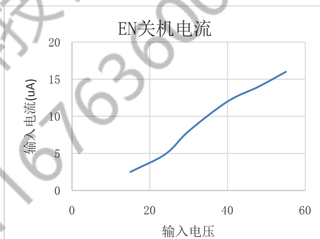
EN 关机电流
