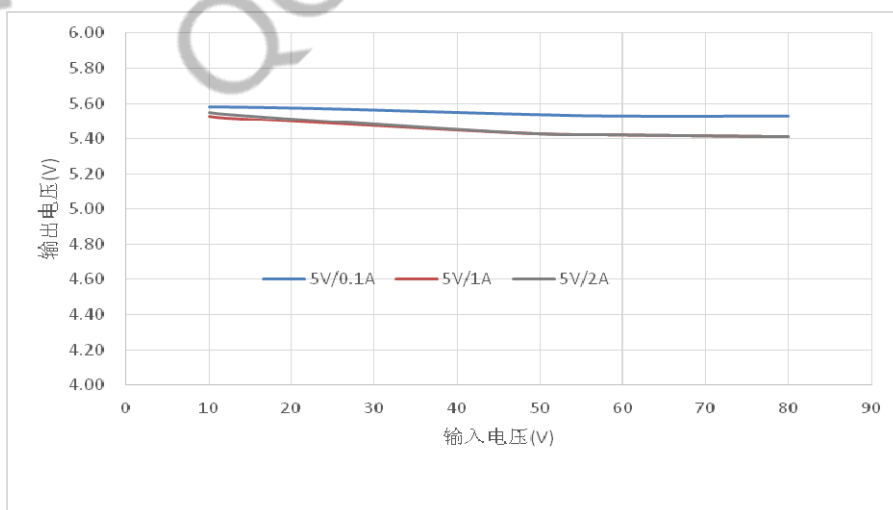
(3) V_O=5V/2A 输出电压与输入电压特性曲线
