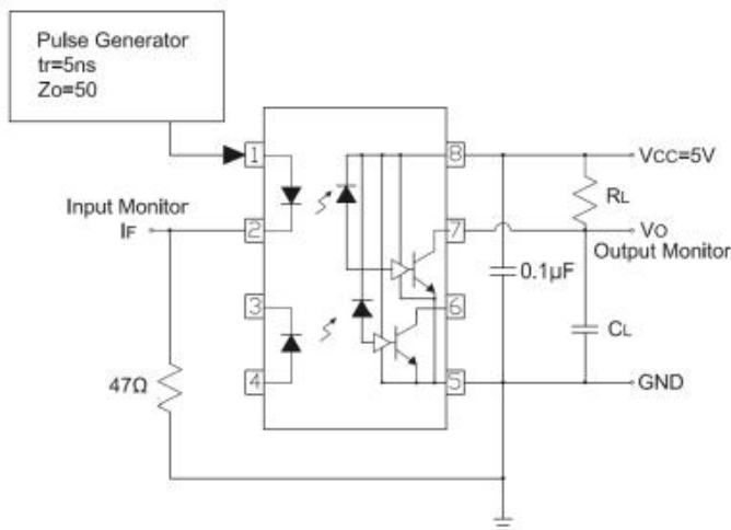
图9: t_{PLH} , t_{PLH} , t_r and t_r 测试电路
