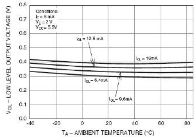
图 2 : V_{OL} VS T_A
