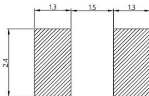
建议焊盘图
