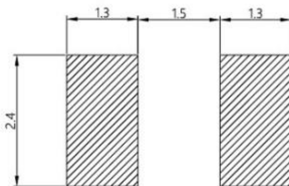
建议焊盘图
