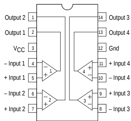
(顶视图)
