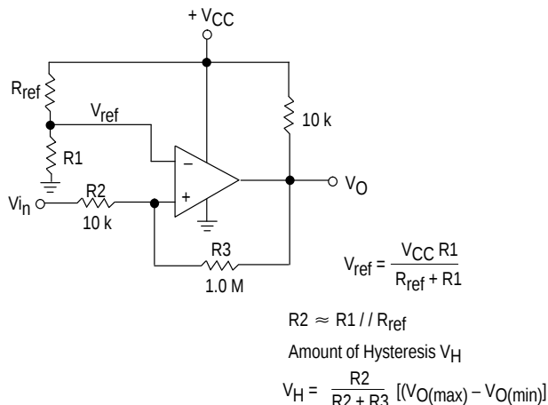
图3 .同相滞后比较器
