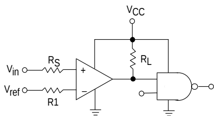
图 6 :驱动逻辑
