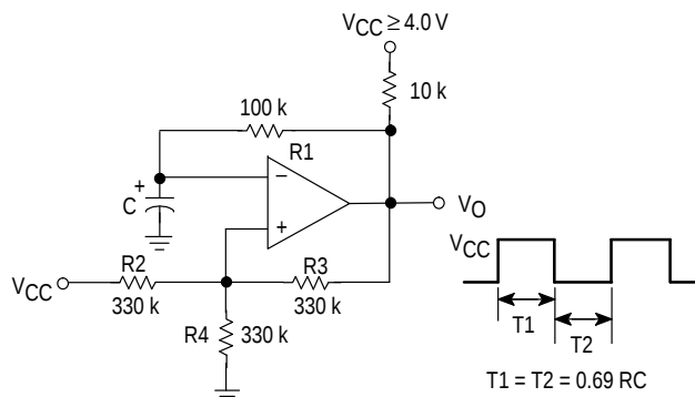
图 7 :方波振荡器
