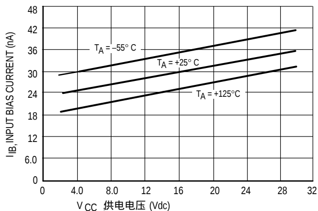
图5 . 输入偏执电流
