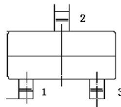
SOT-23-3
