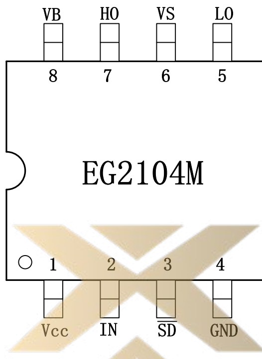
图 4-1. EG2104M 管脚定义
