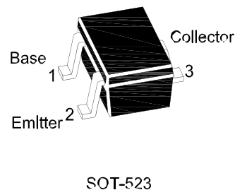
SOT-523
