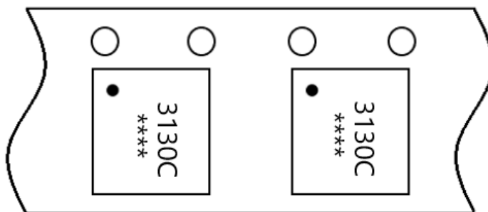
编带示意图
