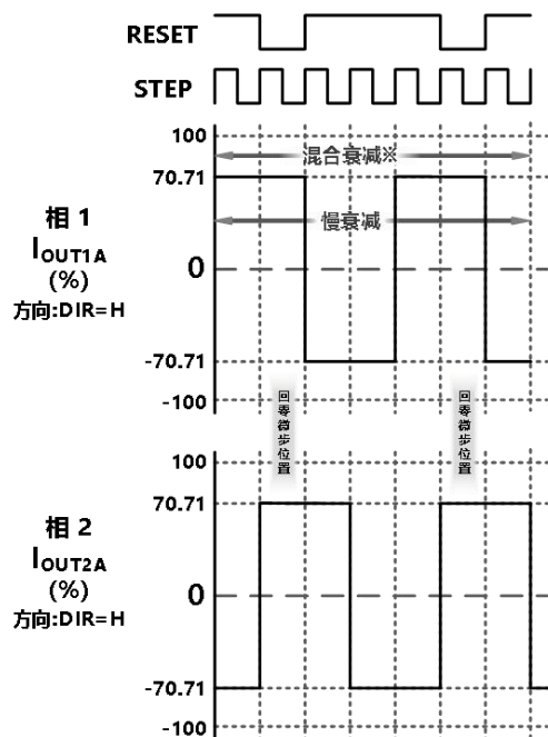
*ROSC引脚接 整步增量衰减模式图
