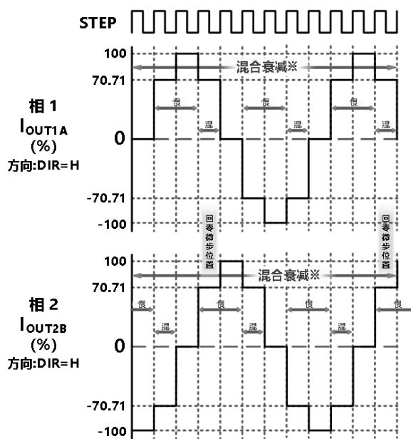
*ROSC引脚接 半步增量衰减模式图
