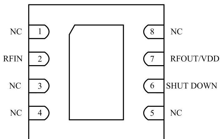
图 2. ATR2037 芯片管脚分布
