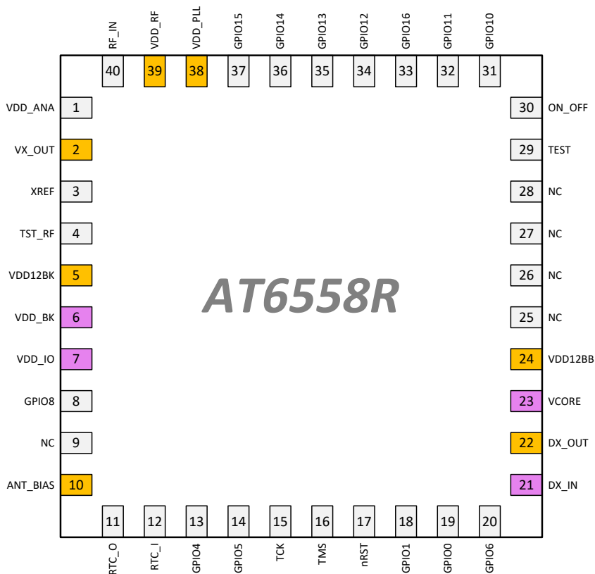
图 2-1 芯片封装管脚排列
