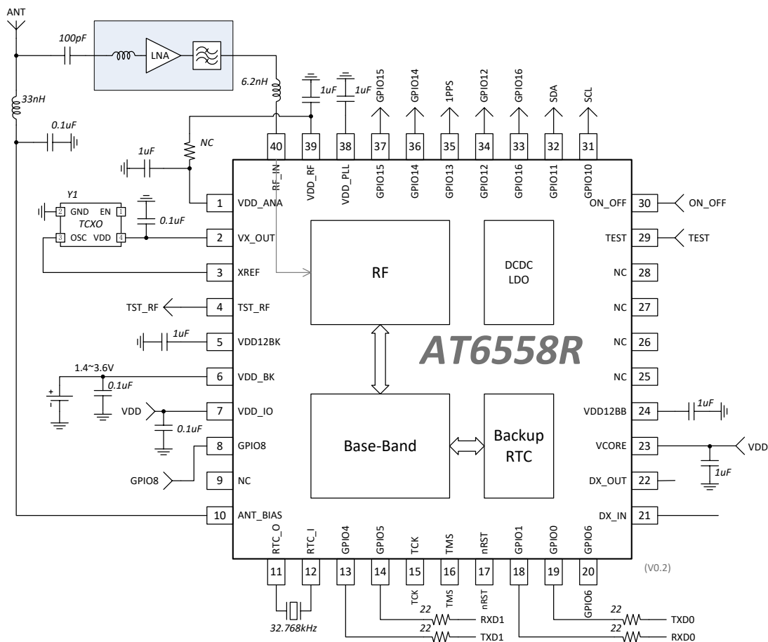
图 5-2 芯片参考设计方案 2（电源直接供电）
