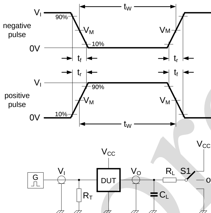
图3 测量开关时间的测试电路
