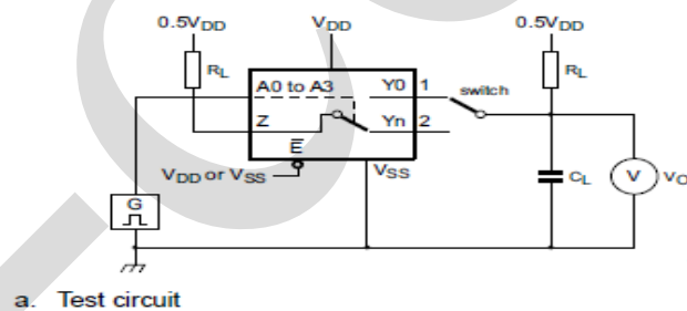
a. Test circuit
