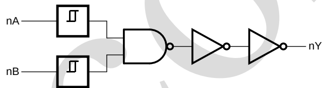
图 2 逻辑框图
