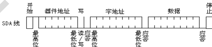
图 8、字节写
