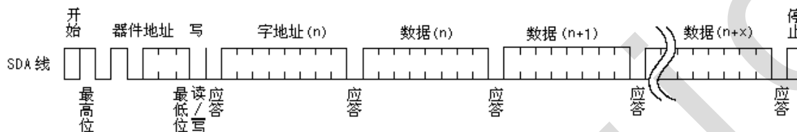
图 9、页写
