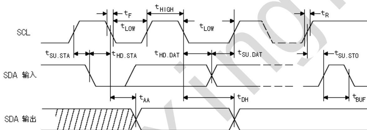
图 5、总线时序
