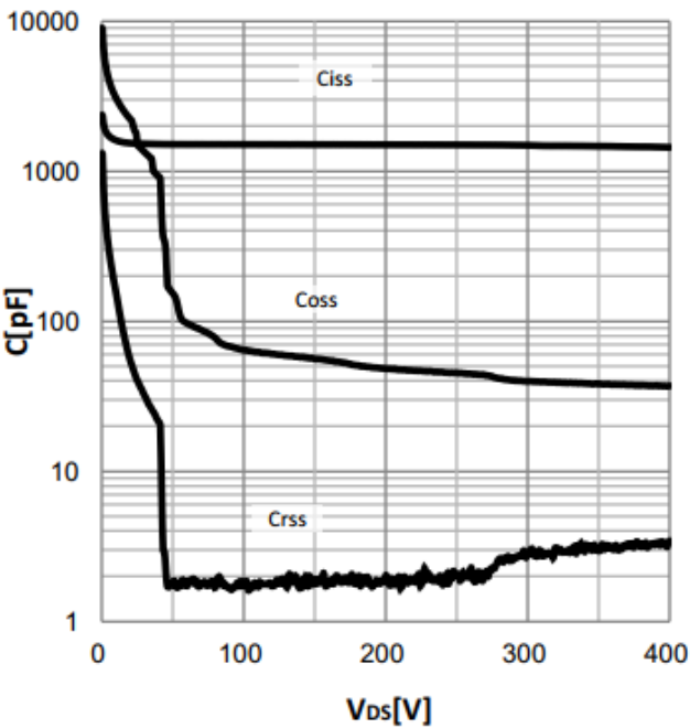
Typ. capacitances
