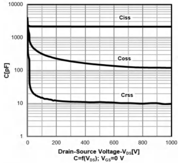
Typ. capacitances
