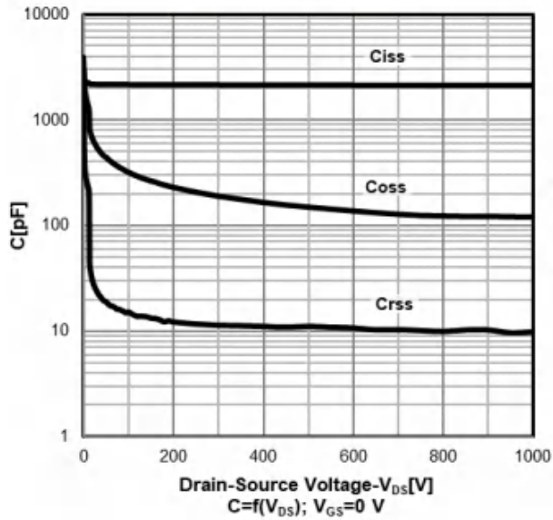
Typ. capacitances
