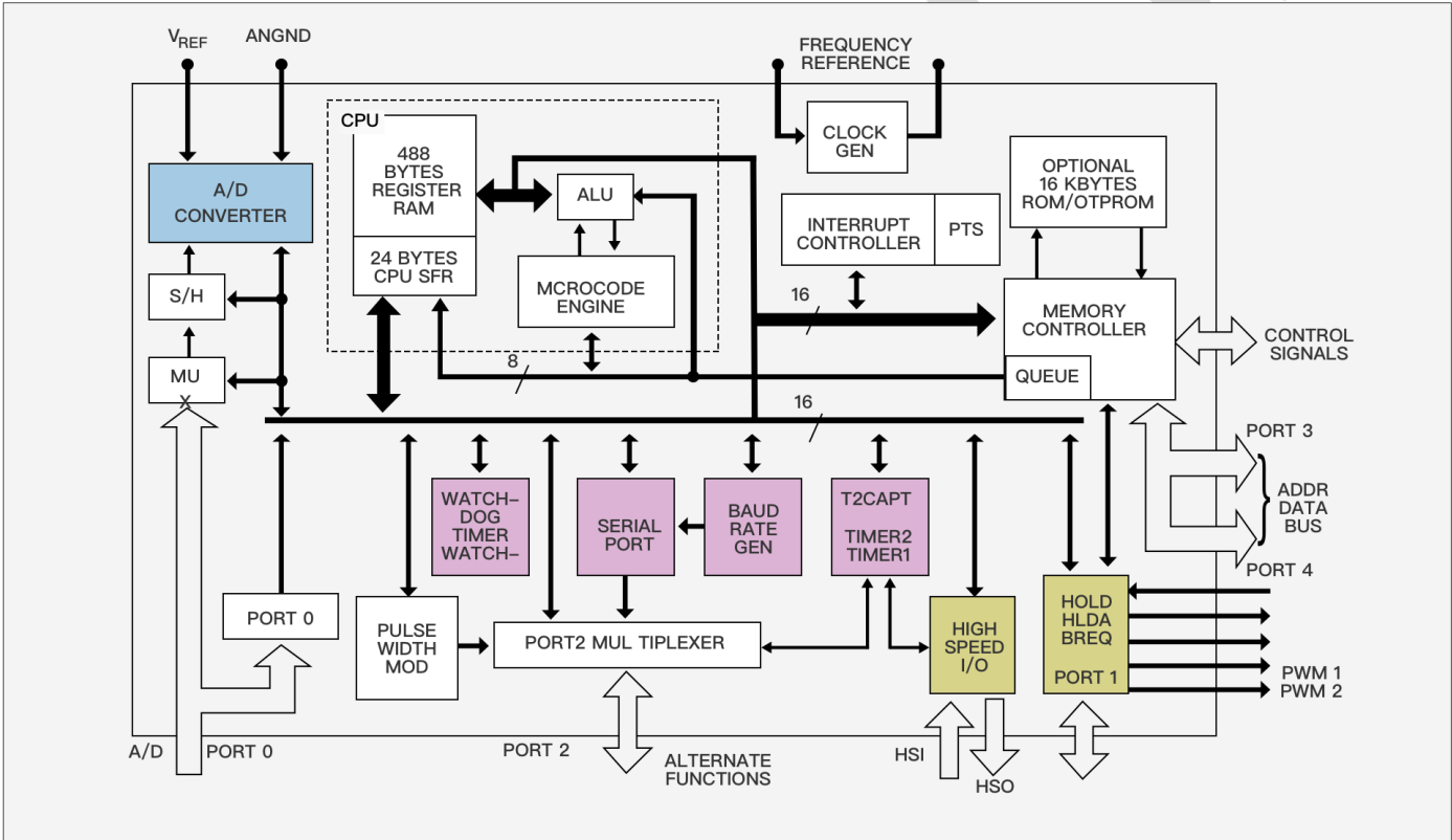
CLM87C196KC20框图
