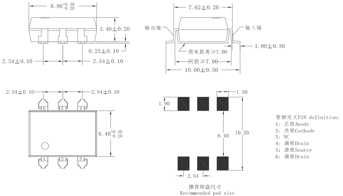
图 9 MT-AQY212FG2S-2 外形尺寸
