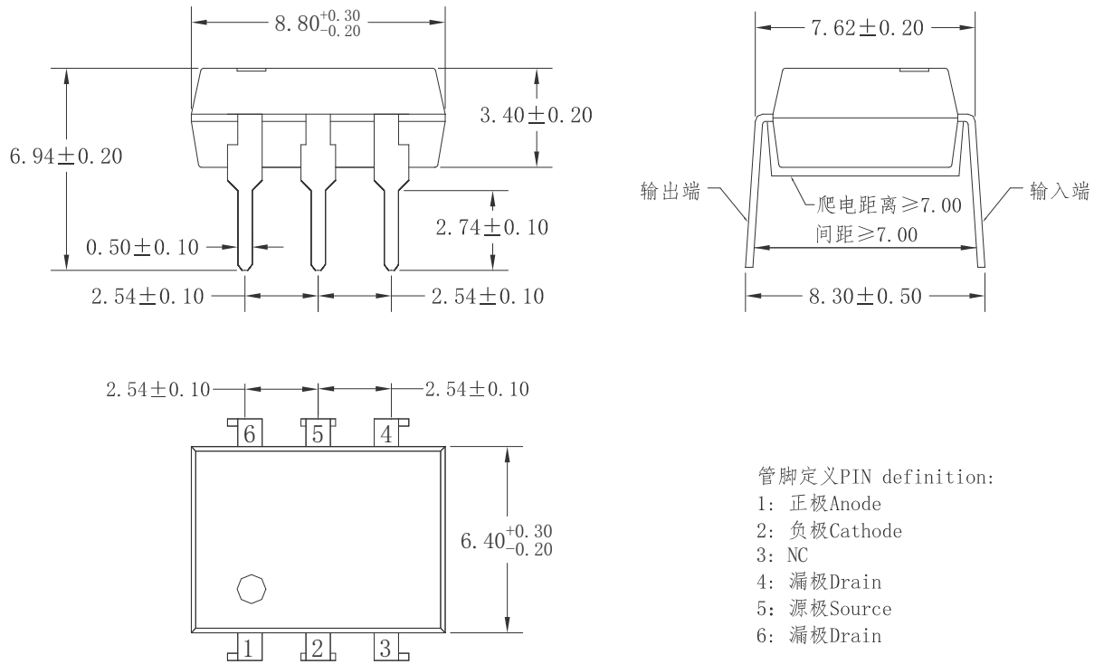
图 8 MT-AQY212FG2S外形尺寸
