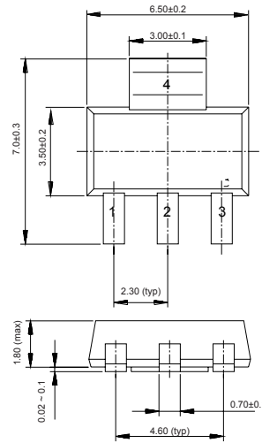
SOT-223
