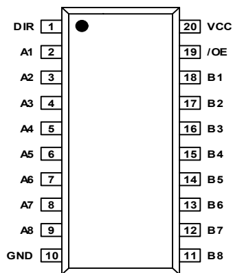
SOP-20/TSSOP-20
