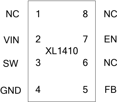
图 2. XL1410 引脚配置
