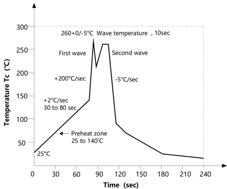
波峰焊温度曲线图 Wave Soldering Profile
